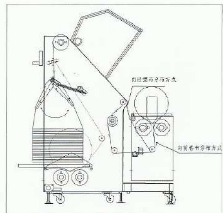
EFC-260功能结构放布图 Functional Structure Layout
