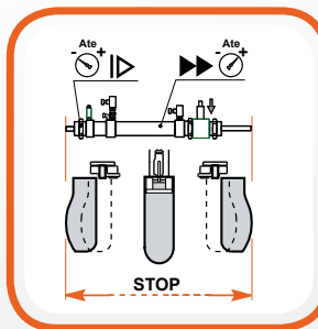
Dispositivo tensione bacino e gamba antistretch, con doppio cilindro per alta velocità e estrema sensibilità per tessuti elasticizzati e blocco meccanico.
